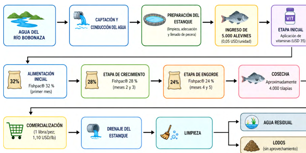
Figura 2. Diagrama de flujo del proceso de cultivo de tilapia en la finca “Tres Chanchitos”
